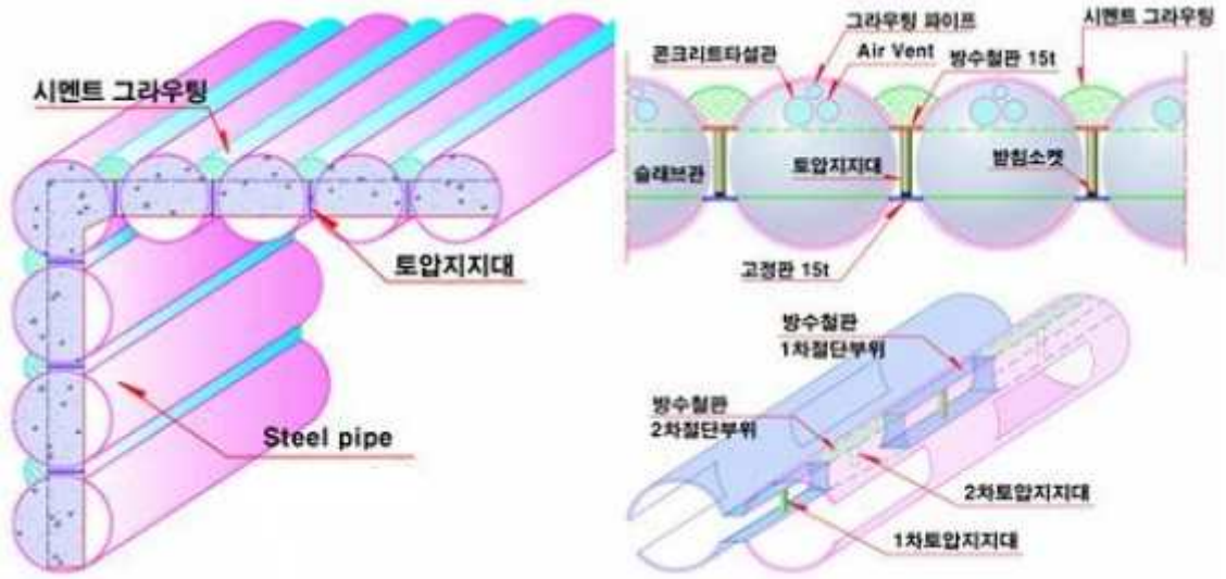
<그림 2> NTR공법
